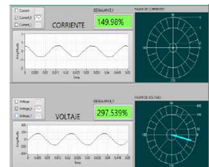
Monitoreo de desbalance de voltaje y corriente.
