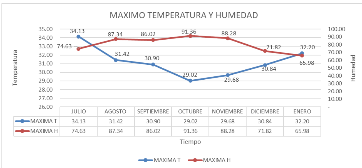
Gráfica 17. Máximos de temperatura y humedad de dormitorio casa bioclimática. Fuente. Elaboración propia.
