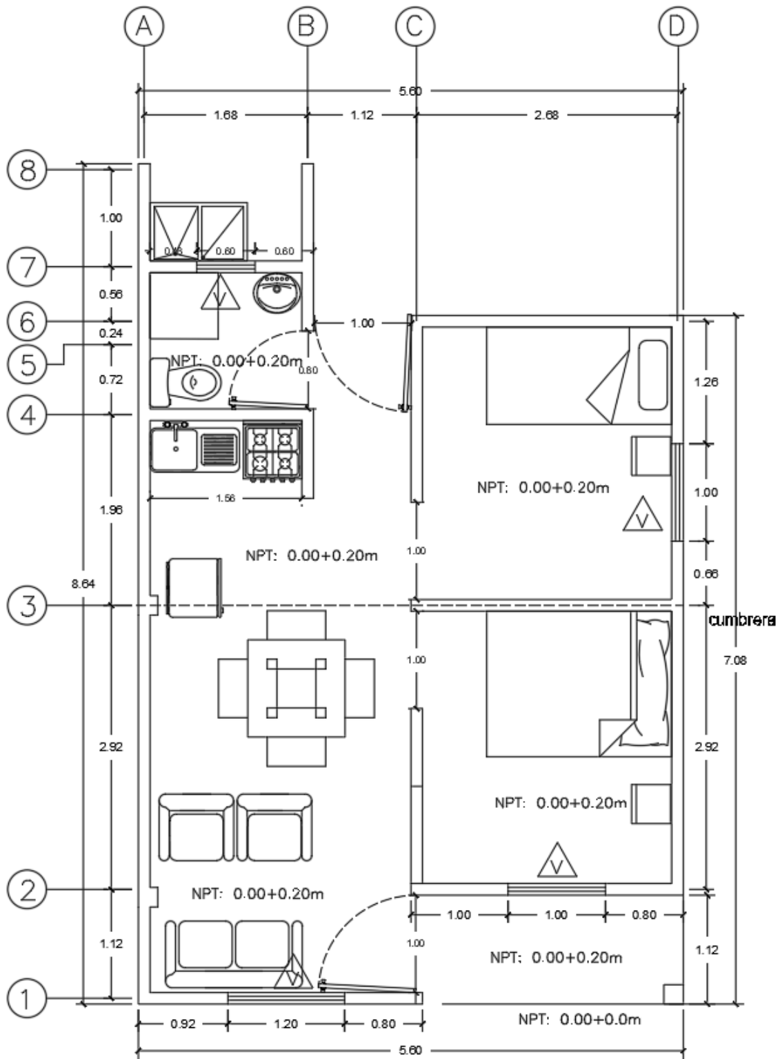
Planta Arquitectonica, vivienda tradicional
