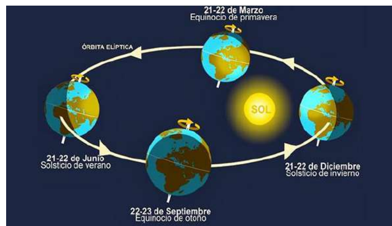
Figura 1. Solsticio de verano y solsticio de invierno. Fuente. Asociación Salvadoreña de Astronomía (ASTRO)
